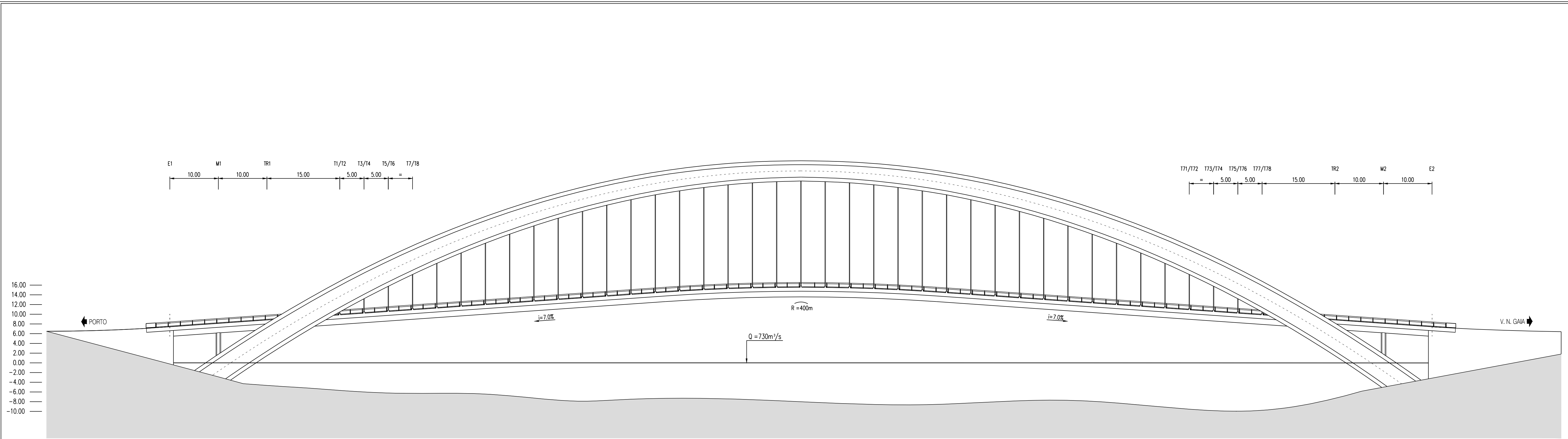
ALÇADO LONGITUDINAL PLANIFICADO
